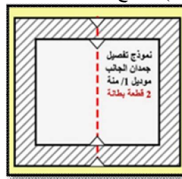
شكل (41) نموذج تفصيل بطانة الجانب ( السلسلة )
