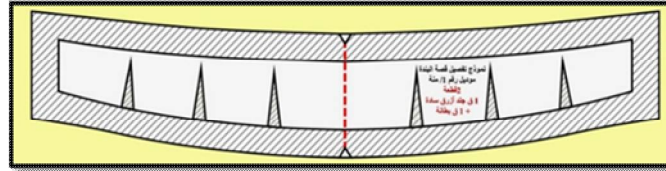
شكل (28) نموذج تفصيل قصة البندة
