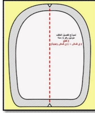
شكل (37) نموذج تفصيل بطانة الخلف
