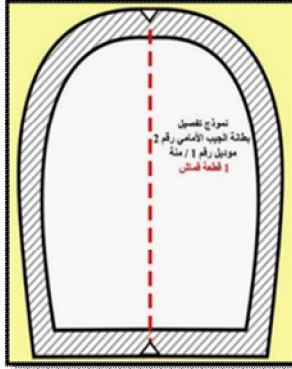
شكل (38) نموذج تفصيل بطانة جيب أمامي رقم (2)
