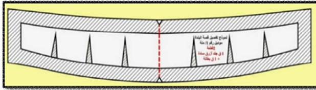
شكل (38) نموذج تفصيل بطانة جيب أمامي رقم (2)
