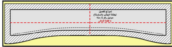
شكل (41) نموذج تفصيل بطانة الجانب ( السلسلة )
